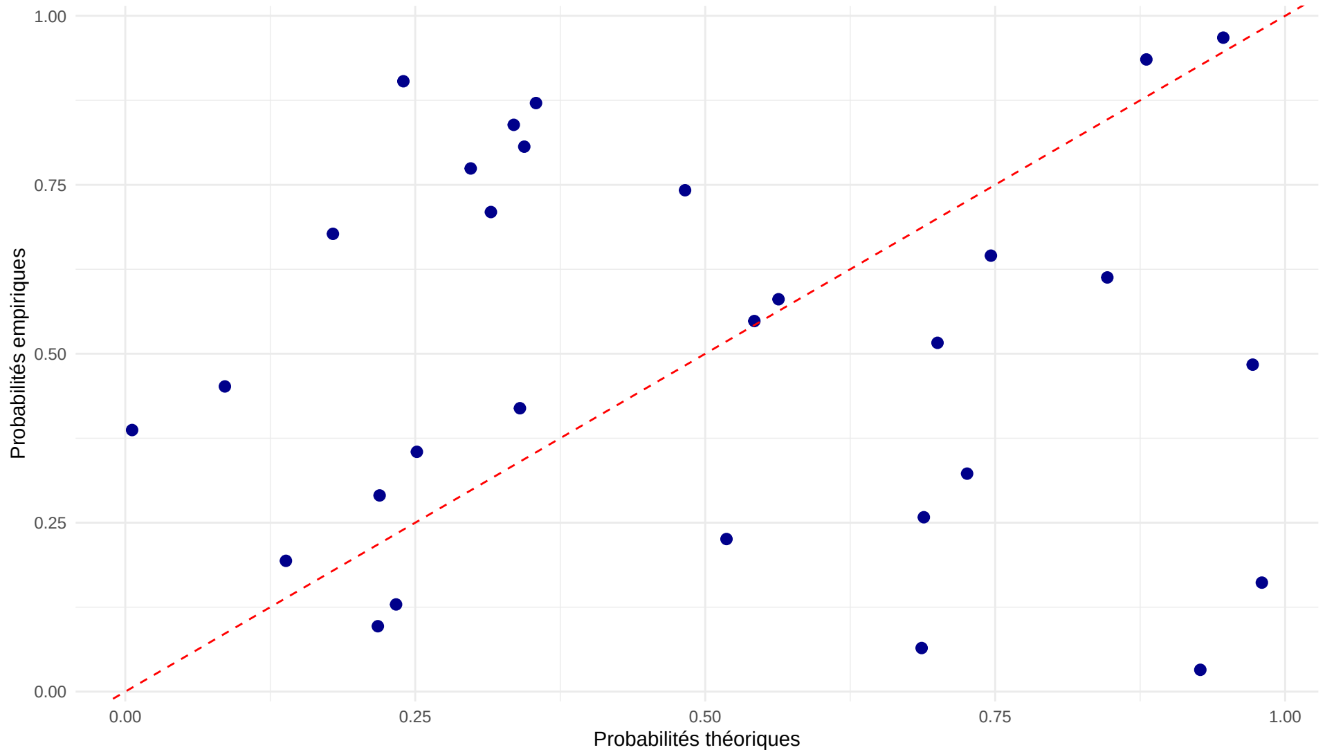
Probability Plot – Modèle GEV non-stationnaire
